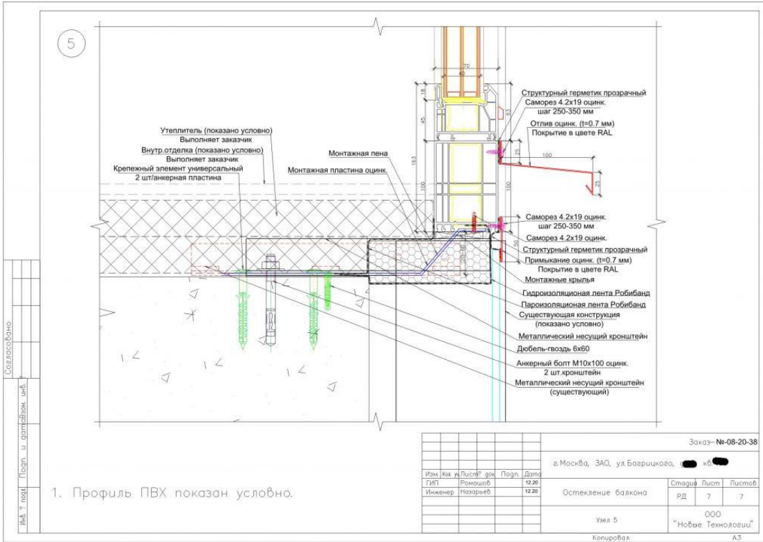
1. Профиль ПВХ показан условно.
